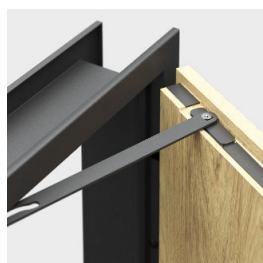
Mecanism de închidere cu arc cu toc din oțel (disponibil în argintiu și negru)
